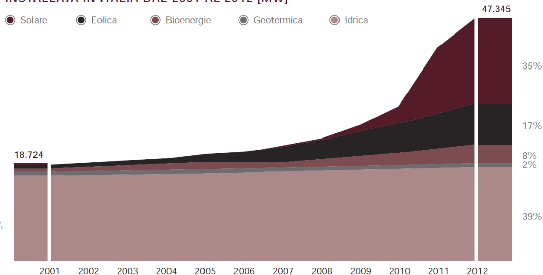
EVOLUZIONE DELLA POTENZA DA FONTI RINNOVABILI INSTALLATA IN ITALIA DAL 2001 AL 2012 [MW]
